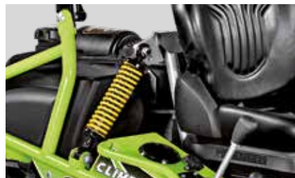
AWD 27 gruppo molla-ammortizzatore
